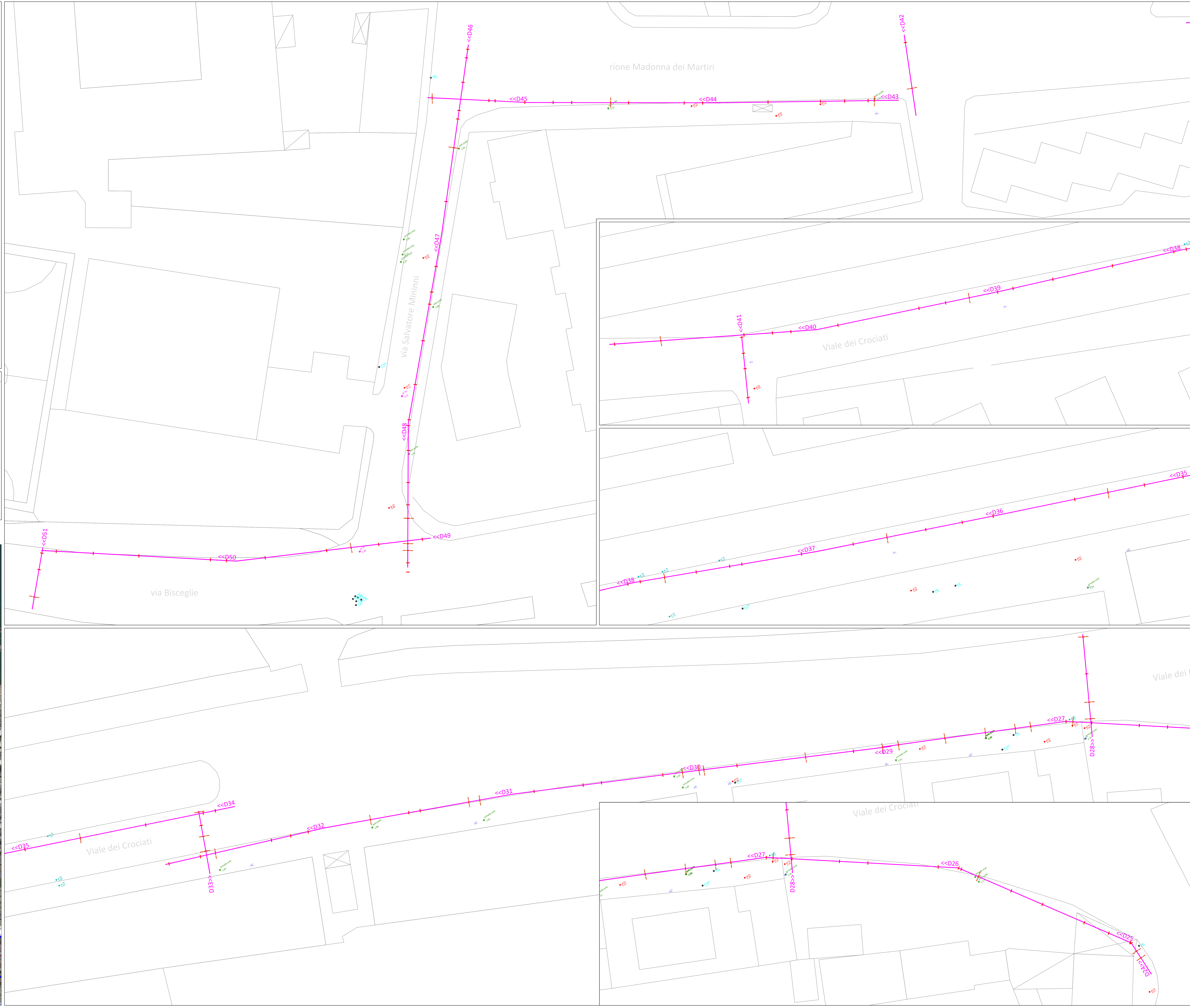
PLANIMETRIA DI INQUADRAMENTO - SCALA 1:5000
