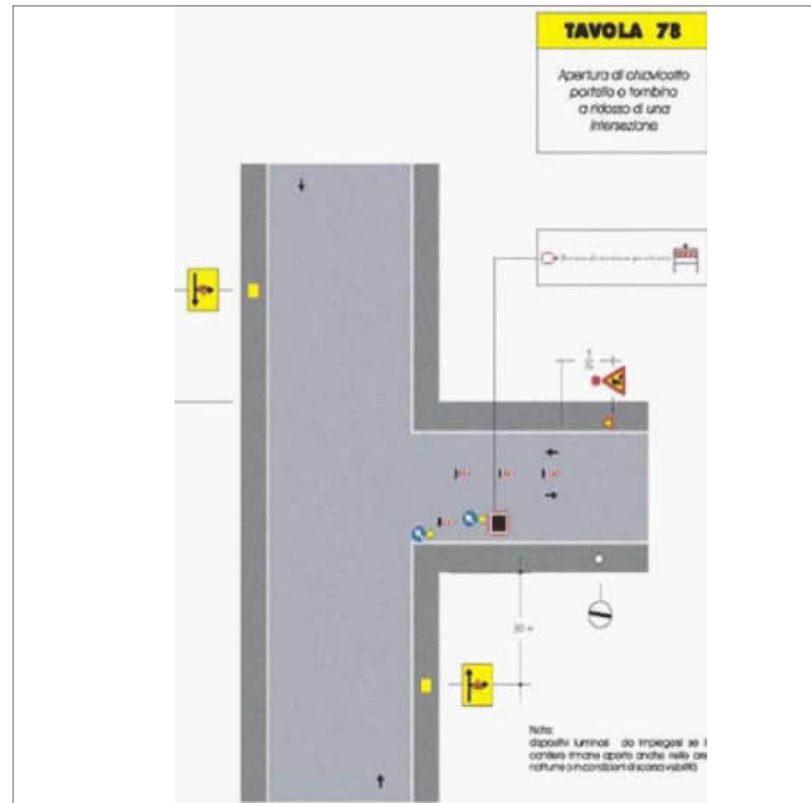
APERTURA CAVIDOTTO A RIDOSSO DI INTERSEZIONE
