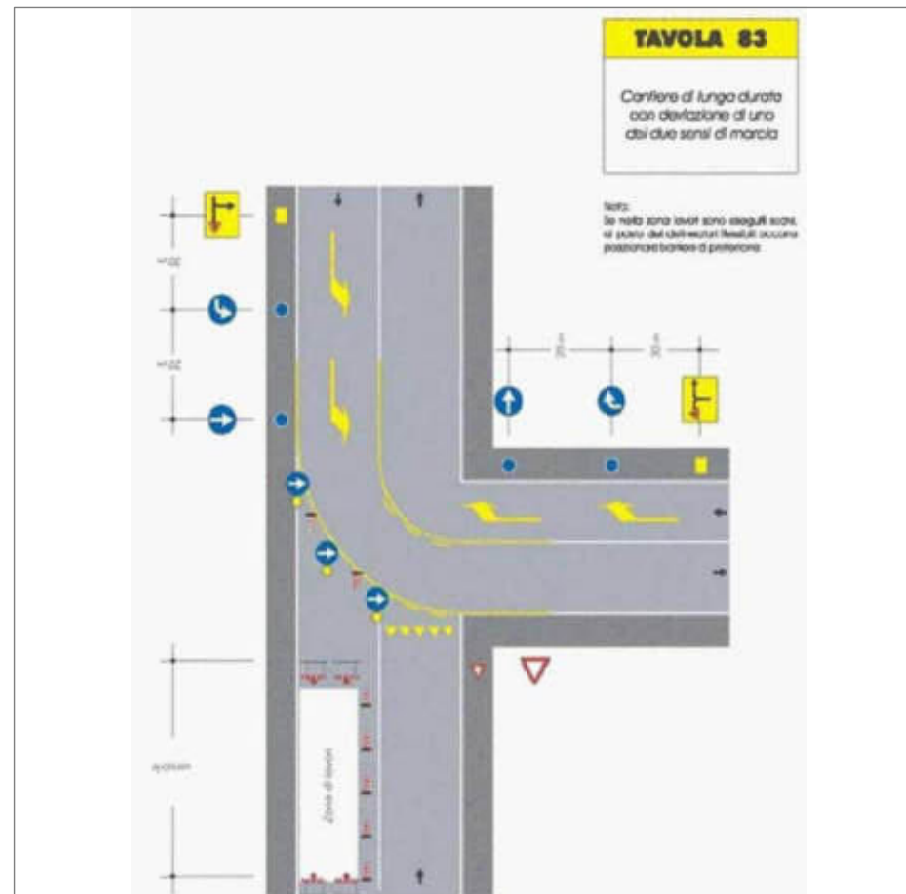
CANTIERE LUNGA DURATA CON DEVIAZIONE
