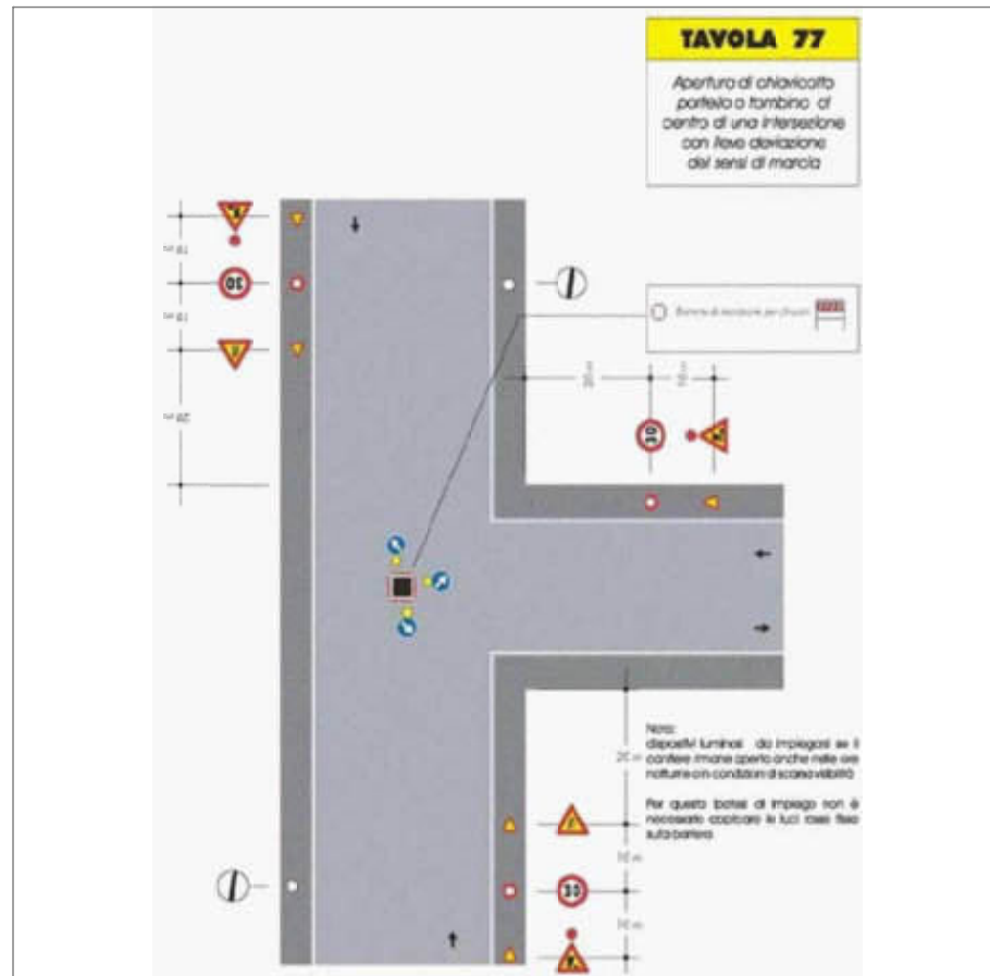
APERTURA CAVIDOTTO AL CENTRO DI INTERSEZIONE
