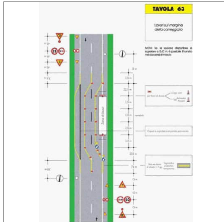
LAVORI SU MARGINE DELLA CARREGGIATA
