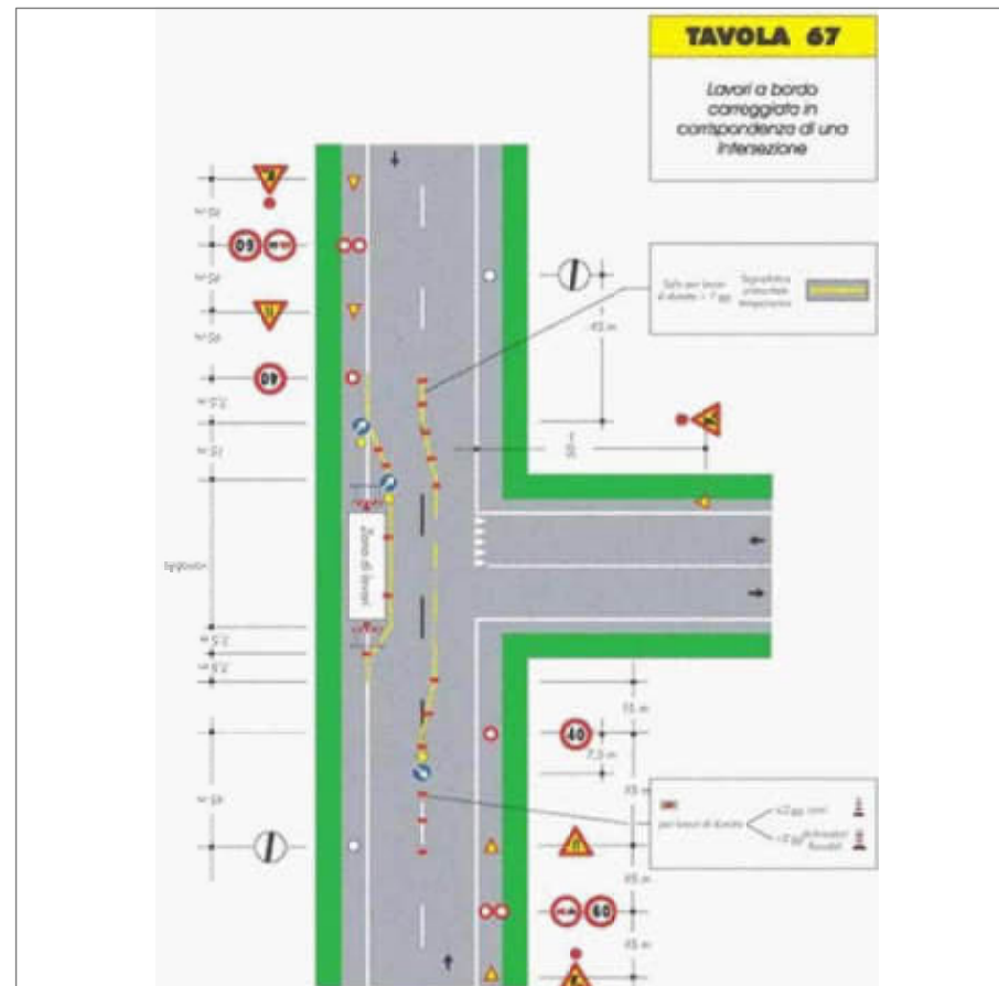
LAVORI A BORDO CARREGGIATA IN CORRISPONDENZA DI UNA INTERSEZIONE
