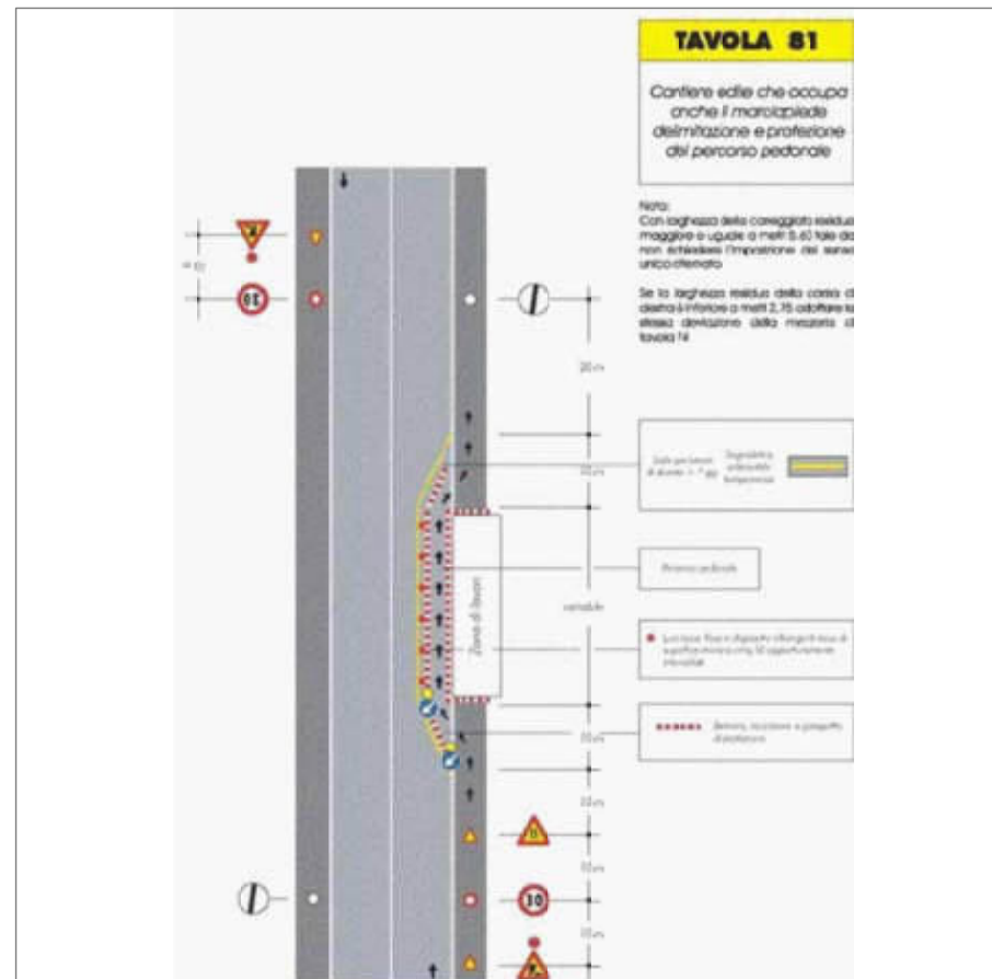
CANTIERE CHE OCCUPA ANCHE MARCIAPIEDE
