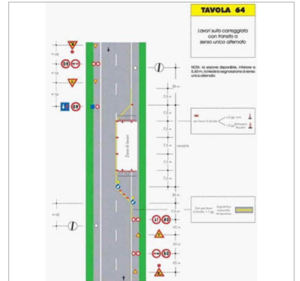
LAVORI SULLA CARREGGIATA CON TRANSITO A SENSO UNICO ALTERNATO
