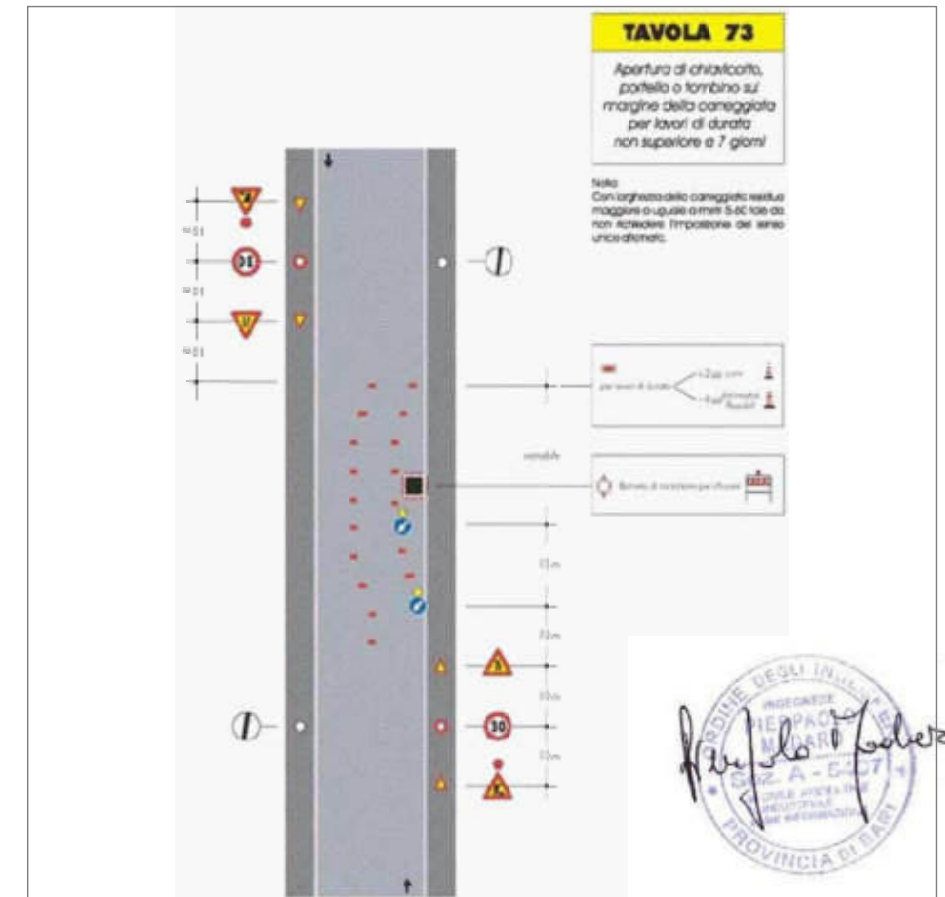
APERTURA CAVIDOTTO O TOMBINO SU MARGINE CARREGGIATA
