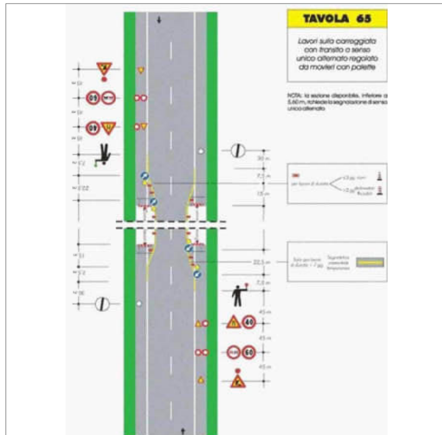
LAVORI SU CARREGGIATA CON SENSO UNICO ALTERNATO
