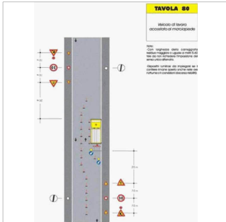
VEICOLO A LAVORO ACCOSTATO AL MARCIAPIEDE
