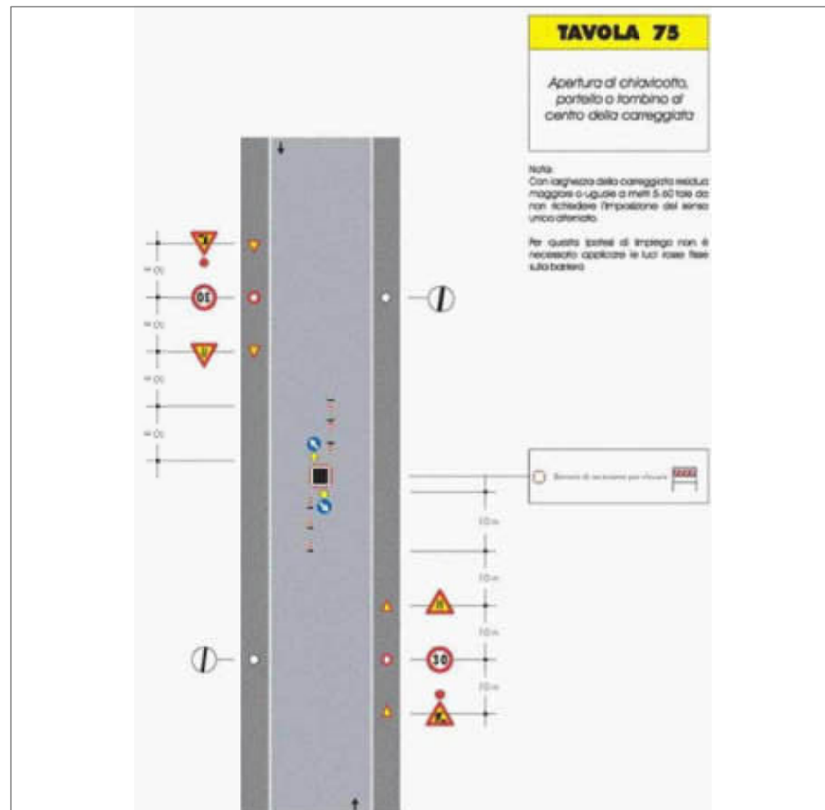
APERTURA CAVIDOTTO A CENTRO CARREGGIATA
