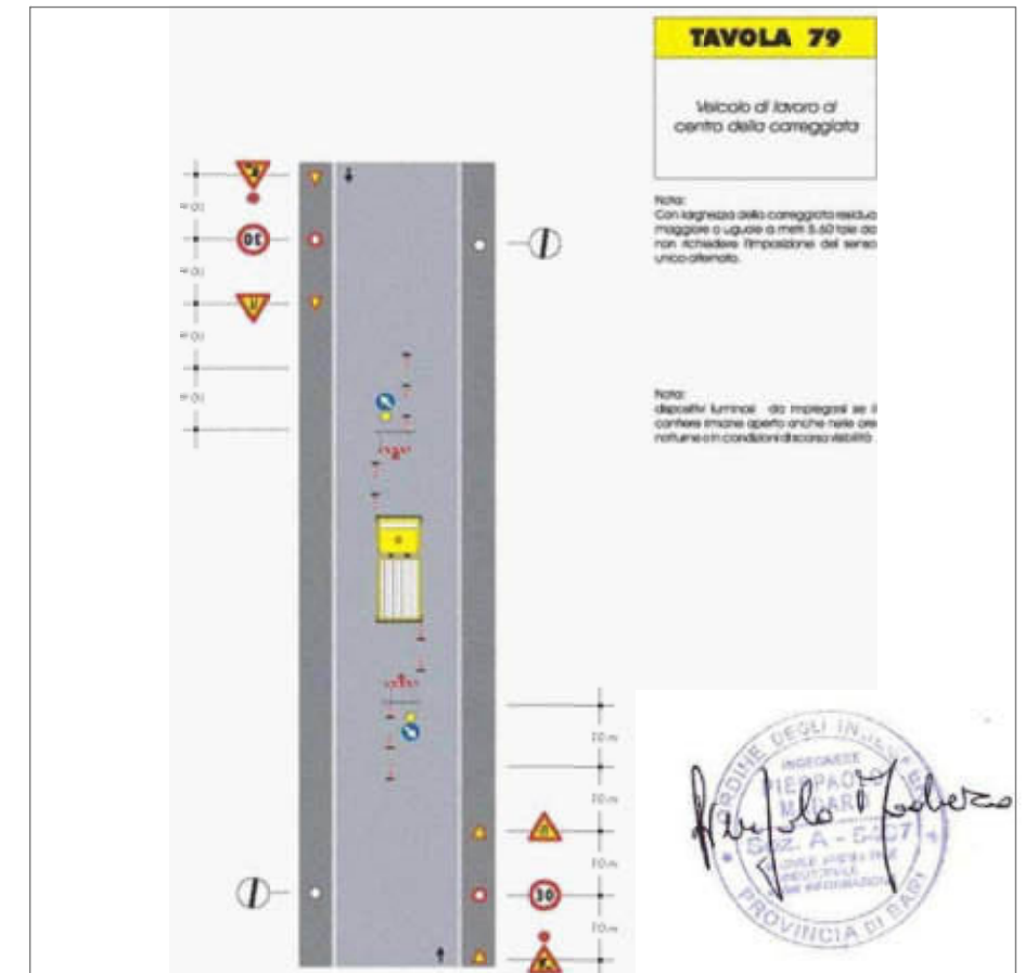
VEICOLO AL LAVORO A CENTRO CARREGGIATA
