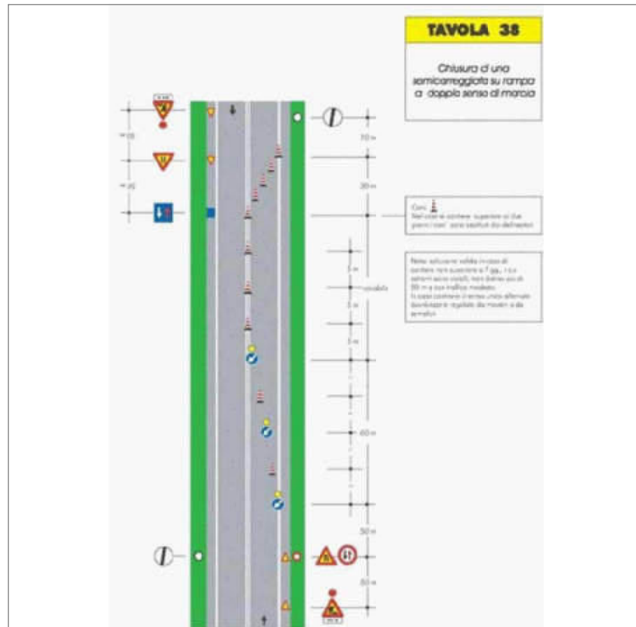
CHIUSURA DI SEMICARREGGIATA
