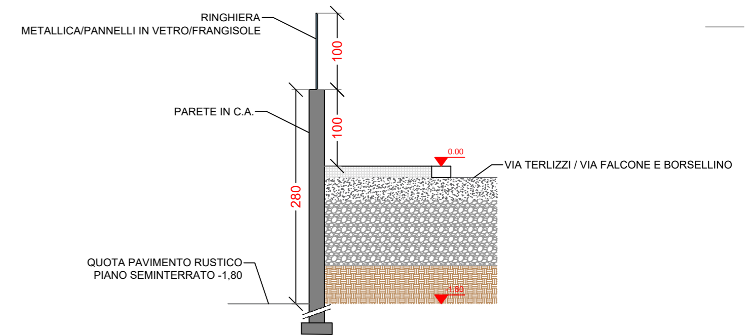
PARTICOLARE COSTRUTTIVO "A" RECINZIONE LATO STRADA SCALA 1:50
