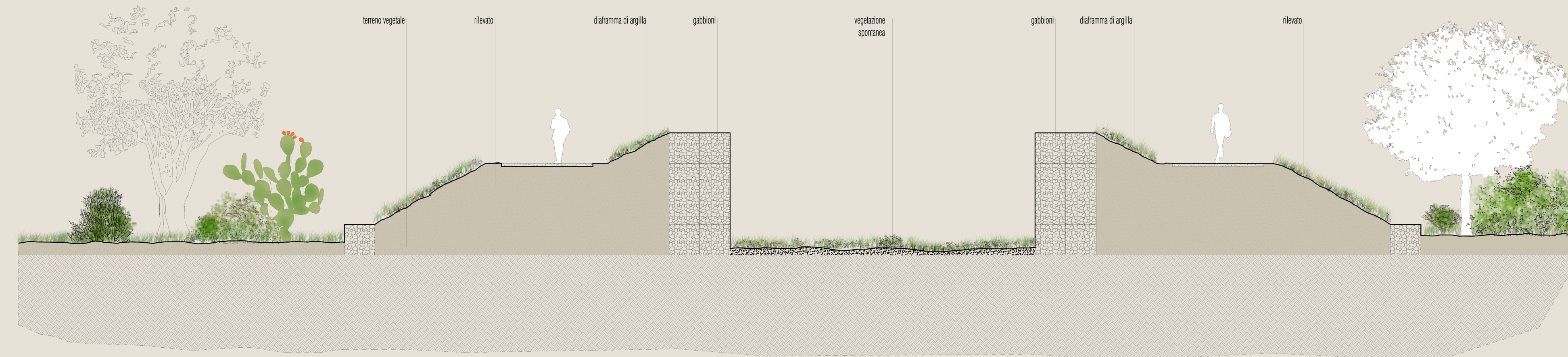
SEZIONE TIPOLOGICA 14
