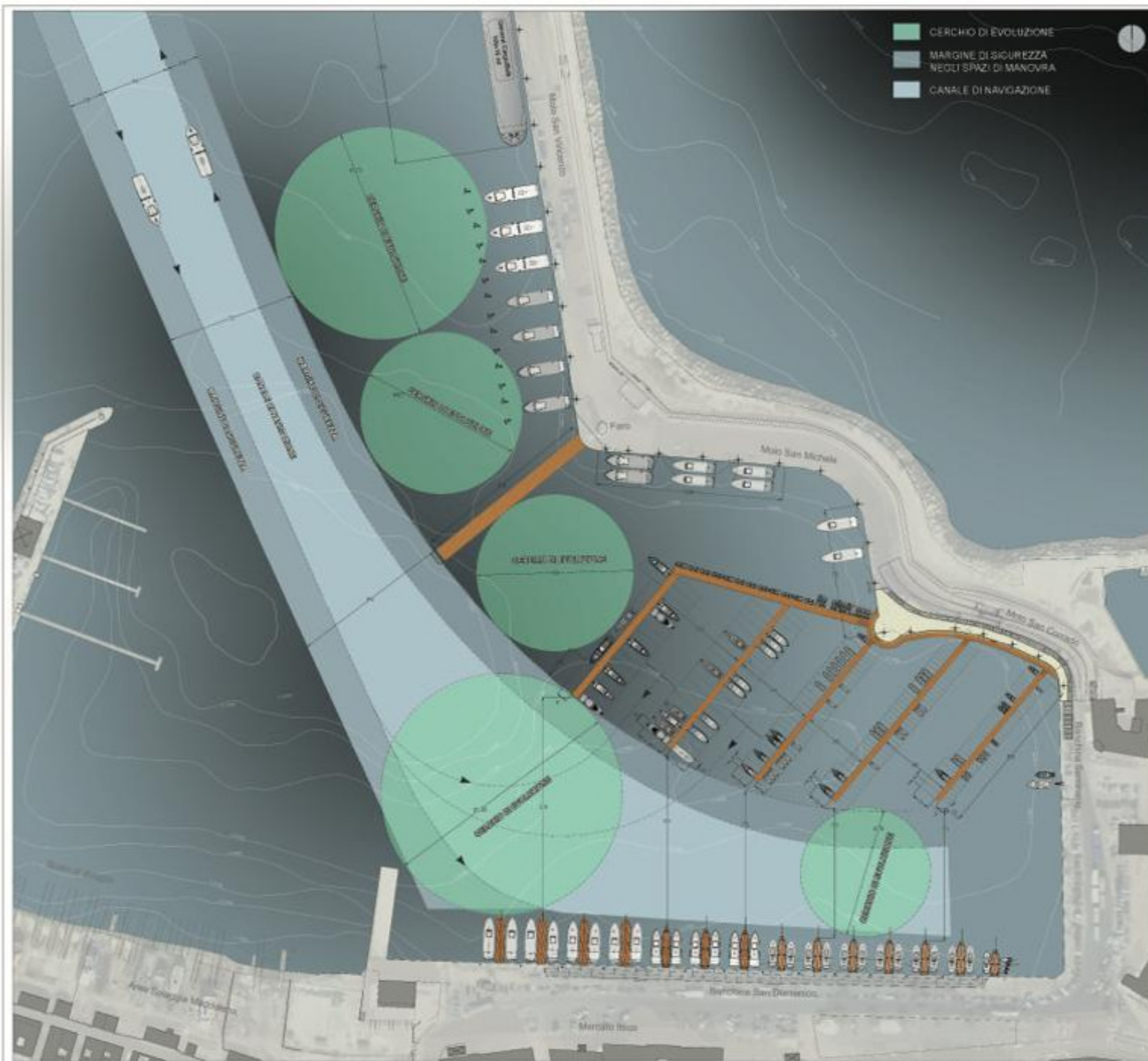
PORTO PESCHERECCIO E NAUTICA DA DIPORTO - NAVIGABILITA' - SCALA 1:1000
