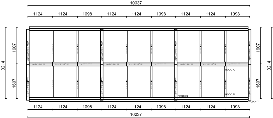
ESECUTIVO TELAIO N.3 - FALDA INCLINATA
