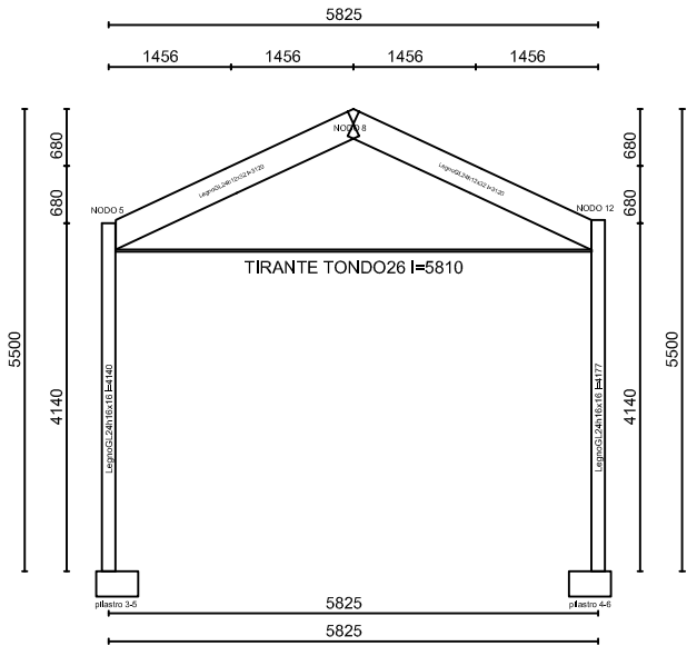
ESECUTIVO TELAIO N.2
