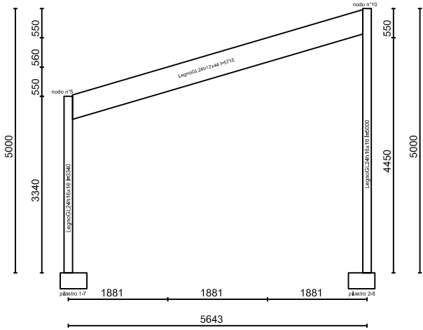
ESECUTIVO TELAIO N.1
