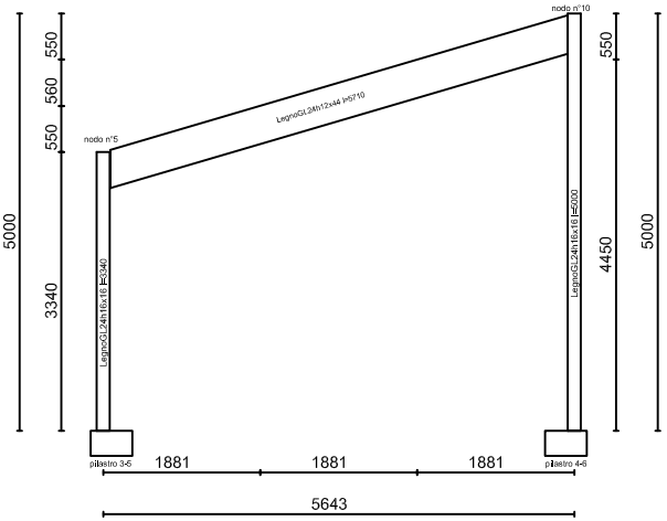
ESECUTIVO TELAIO N.2
