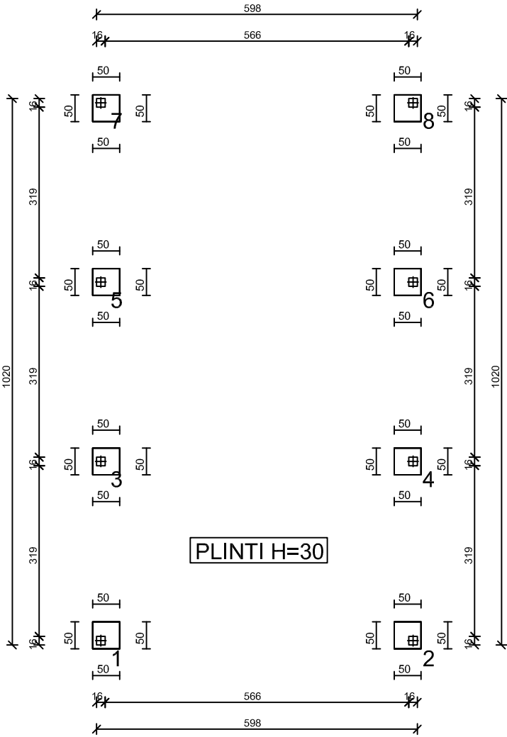
PIANTA FONDAZIONI
