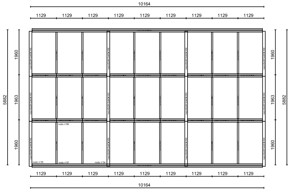
ESECUTIVO TELAIO N.15 - falda inclinata
