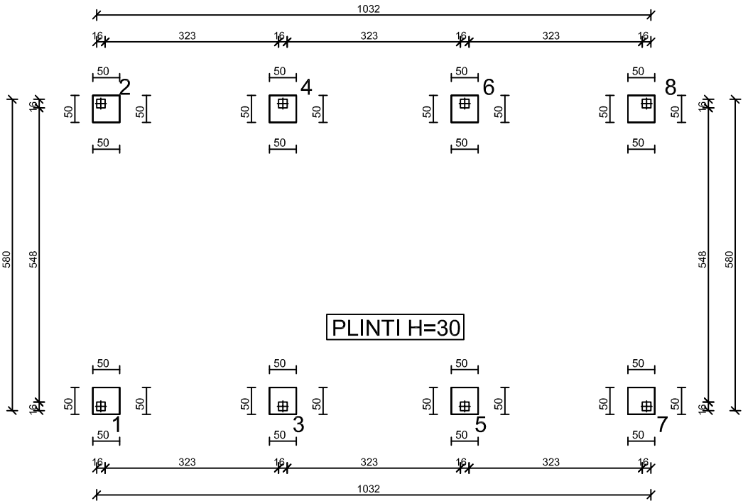
PIANTA FONDAZIONI
