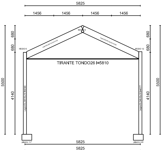
ESECUTIVO TELAIO N.1
