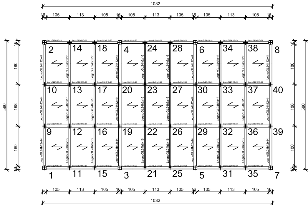
PIANTA IMPALCATO QUOTA m: 5.00 SCHEMA DEI CARICHI - SOLAIO: PERLINATO s=3cm
