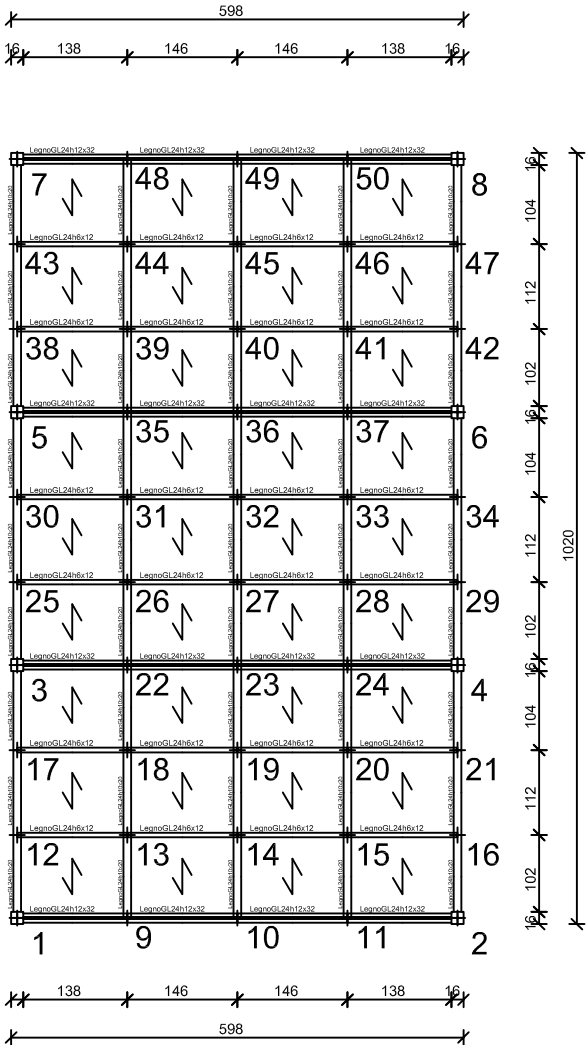
PIANTA IMPALCATO QUOTA m: 5.50 SCHEMA DEI CARICHI - SOLAIO: PERLINATO s=3cm
