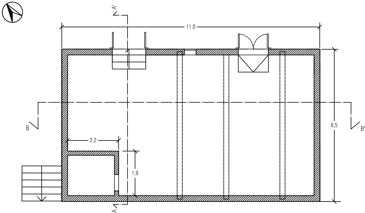
Pianta
