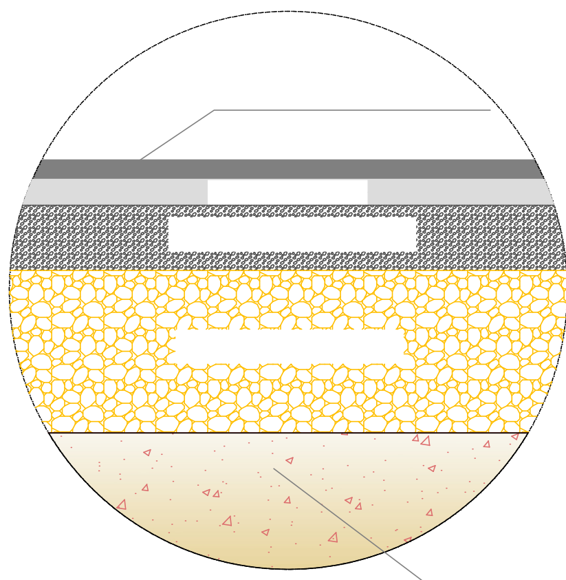
PARTICOLARE 1 PACCHETTO STRADALE
